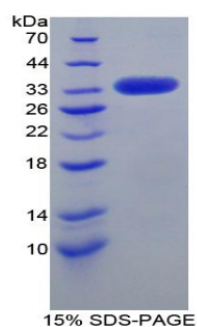
15% SDS-PAGE
