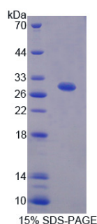
15% SDS-PAGE
