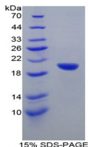
15% SDS-PAGE
