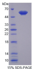
15% SDS-PAGE
