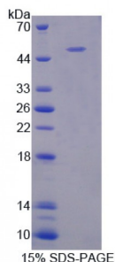
15% SDS-PAGE
