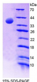
15% SDS-PAGE
